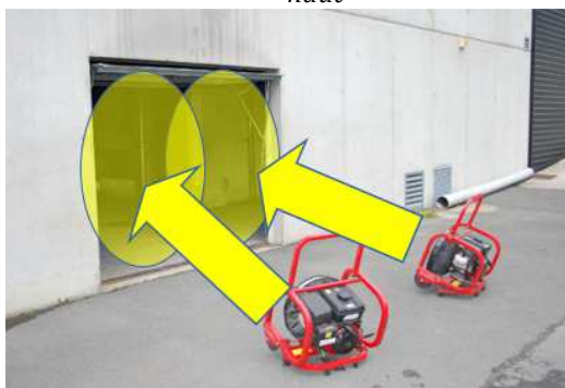
Illustration n°4 : Utilisation de deux ventilateurs en V (l'un vers le bas de l'ouvrant, l'autre, vers le haut)
