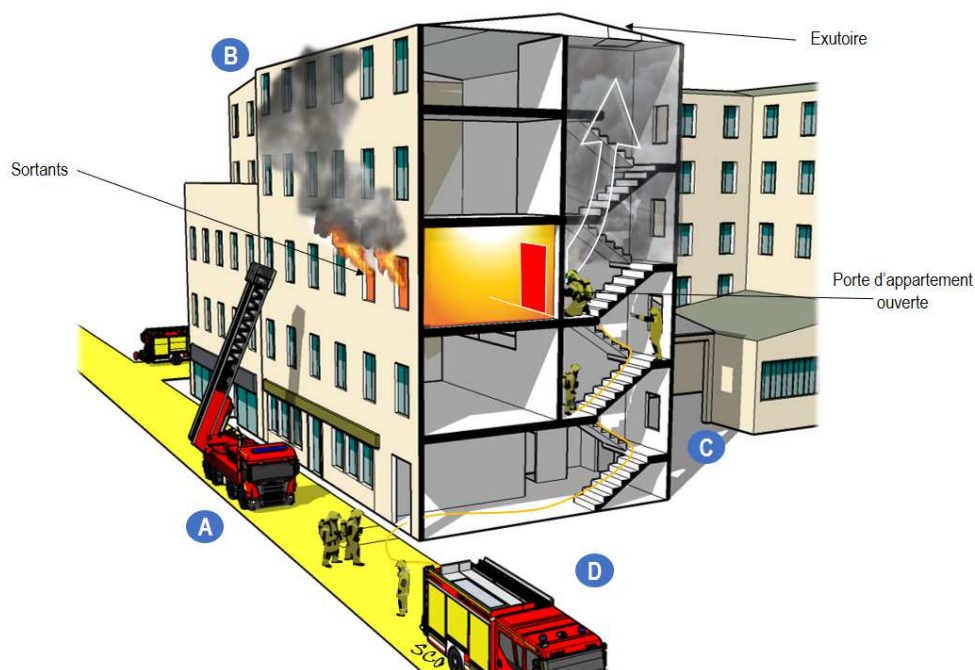
Etape n°1 : le feu se développe et les fumées se répandent dans la cage d'escalier
