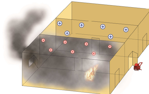
Etape n°2 : Le local contigu à protéger est mis en surpression
