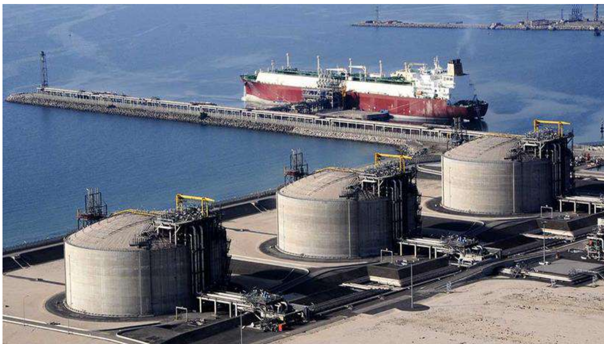
Terminal méthanier de Fos Cavaou à Fos-sur-Mer © Gaz-Mobilité
