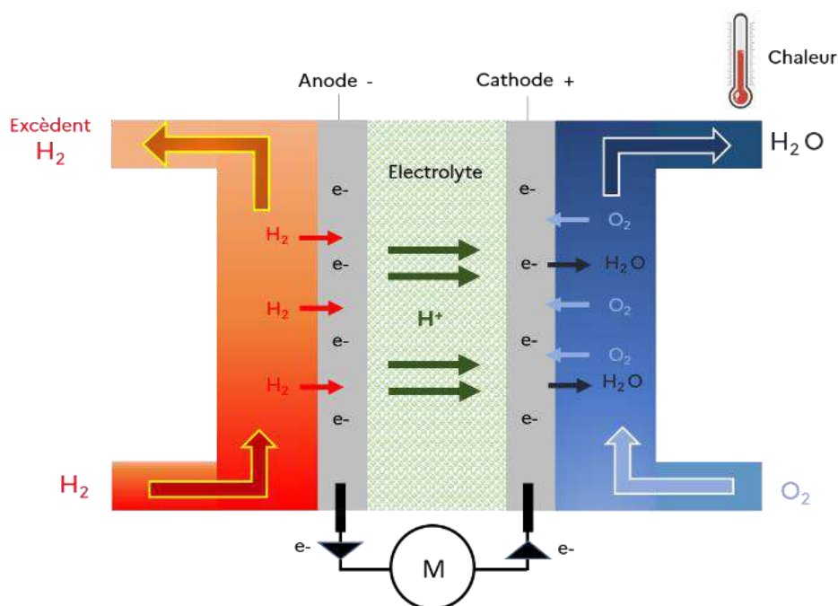
Principe de fonctionnement d'une pile à hydrogène © Christophe Perdrisot - DGSCGC
