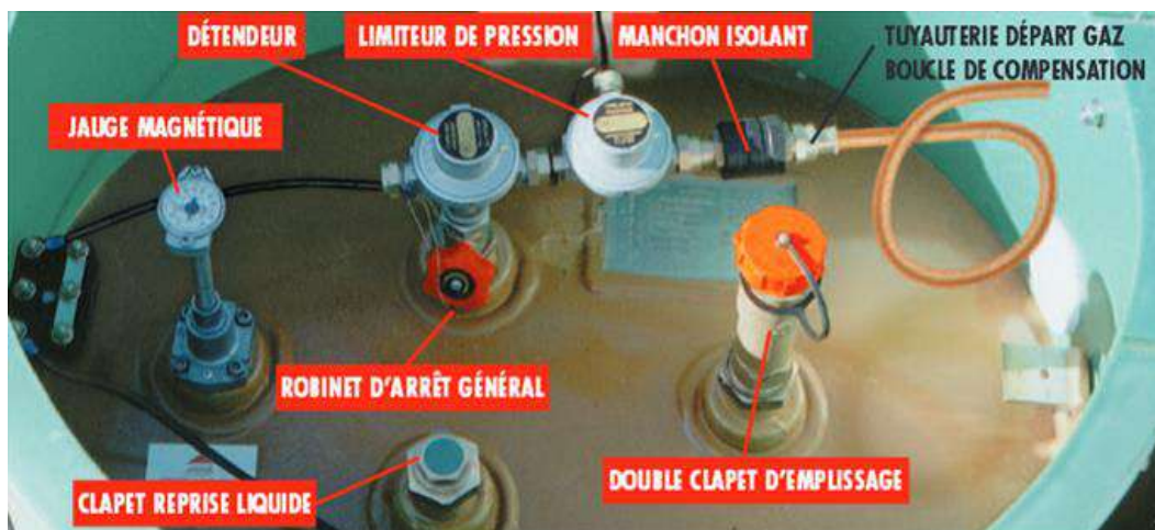
Organe de coupure (robinet d'arrêt général) sur une citerne enterrée. © www.vitogaz.com
